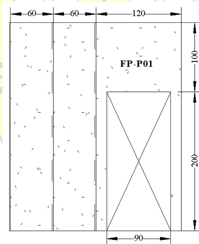
Bukaan Pintu 2 Model 2
