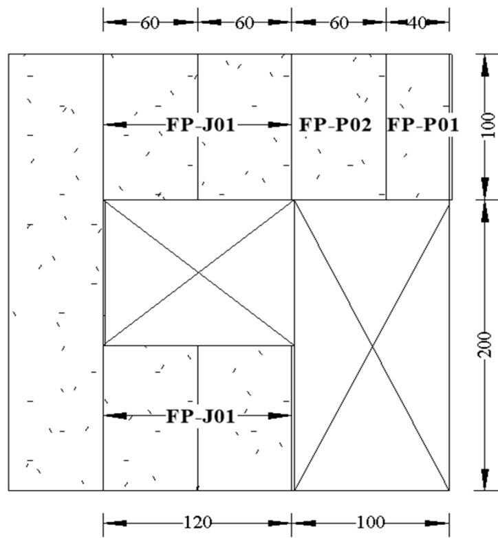
Bukaan Pintu 1 model 1
