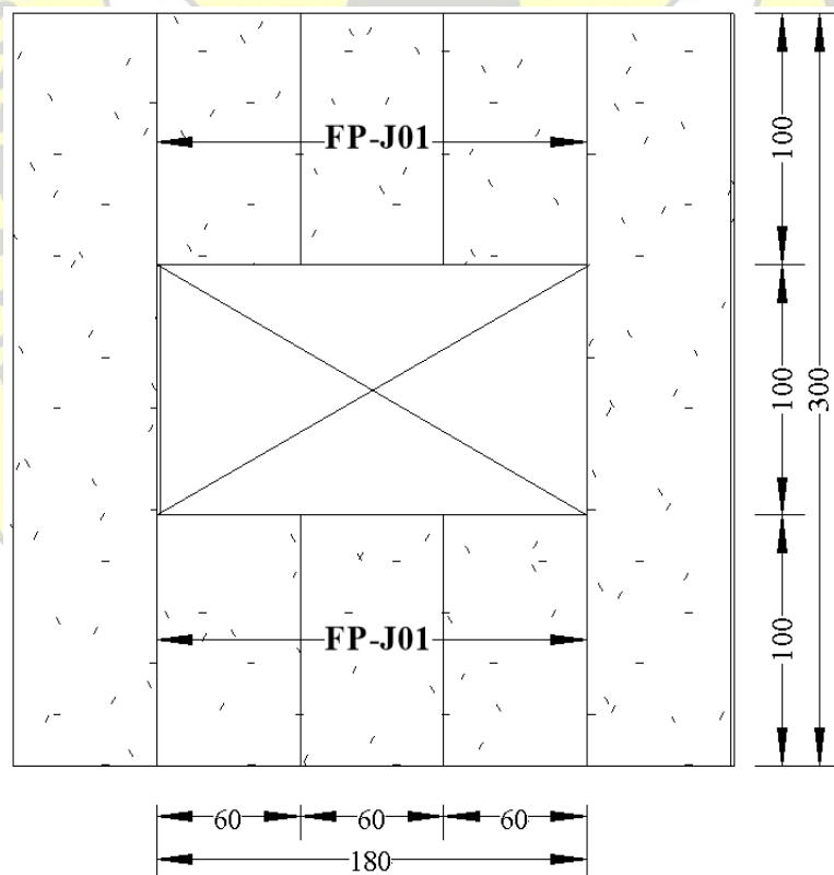
Bukaan Jendela 3 Daun
