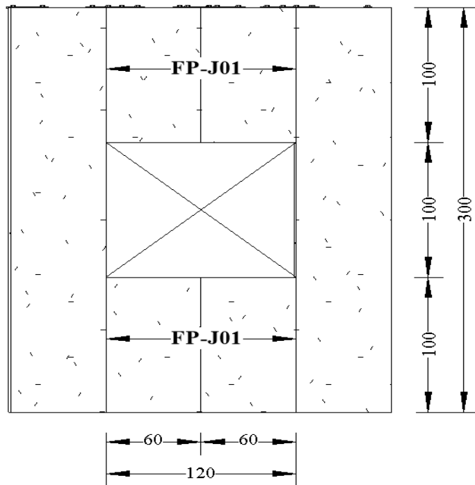
Bukaan Jendela 2 Daun
